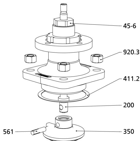
Fig. 12: Montaje del obturador y el vástago
