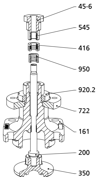
Fig. 10: Montaje de la junta con perfil en V de PTFE
