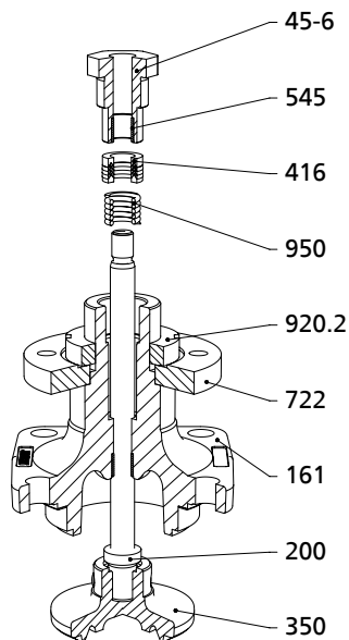
Fig. 7: Desmontaje de la junta con perfil en V de PTFE
