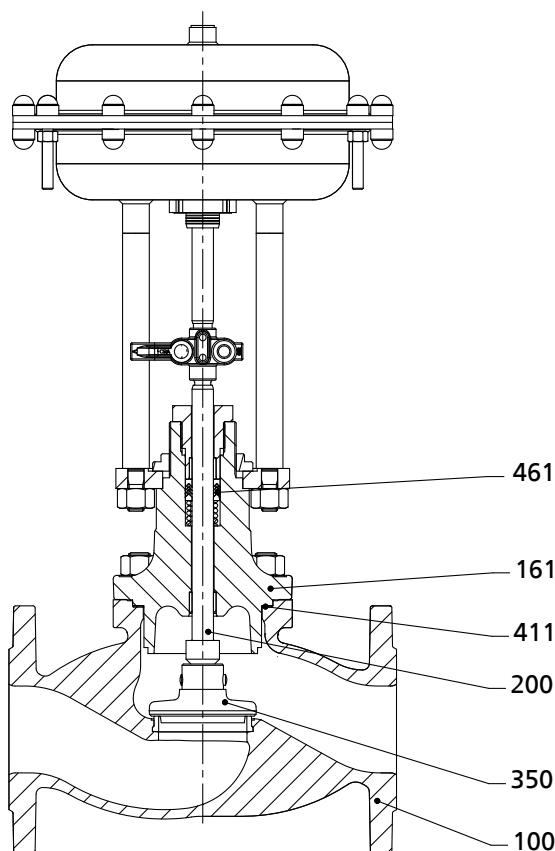
Fig. 5: Vista de sección
