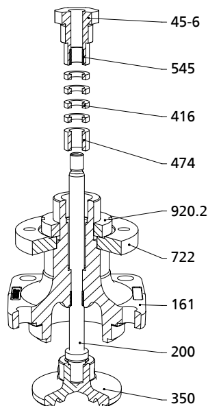
Fig. 11: Montaje de la empaquetadura del prensaestopas de grafito
