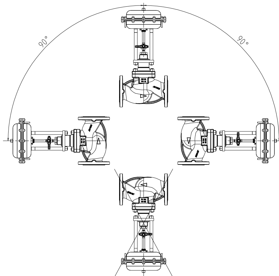
Fig. 6: PA-N 300 a PA-N 540
