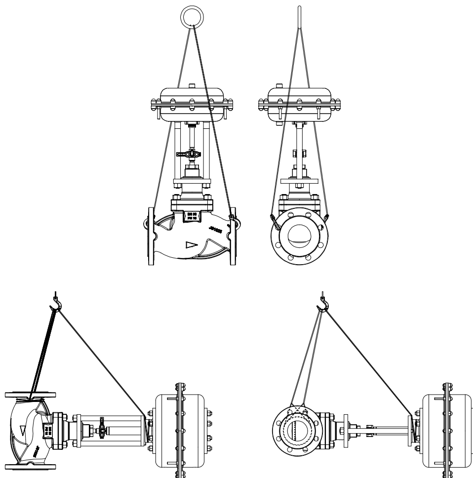
Fig. 1: Transporte de la válvula con actuador neumático
