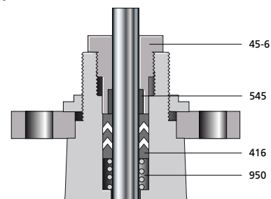
Junta con perfil en V de PTFE
