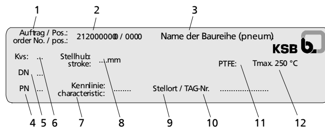
Fig. 4: Placa de características de la válvula (ejemplo)
