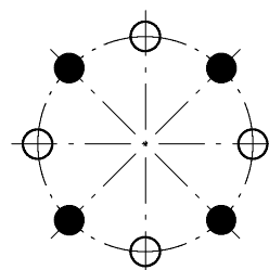
DN 65 PN 10/16 (acero/hierro fundido): DIN EN 1092-1 con DIN EN 1092-2: círculo con orificios DIN EN 1092-1 girado 22,5°, 4 orificios roscados, 4 orificios libres
