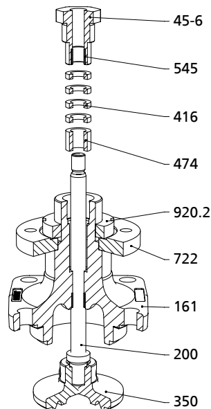
Fig. 8: Desmontaje de la empaquetadura del prensaestopas de grafito
