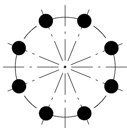
DN 65 PN 10/16 (acero/acero): DIN EN 1092-1 con DIN EN 1092-1: 8 orificios roscados
