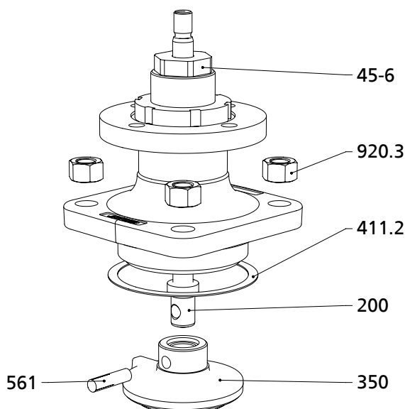
Fig. 9: Desmontaje del obturador y el vástago
