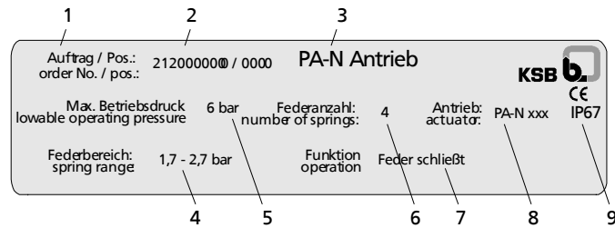
Fig. 3: Placa de características del actuador (ejemplo)
