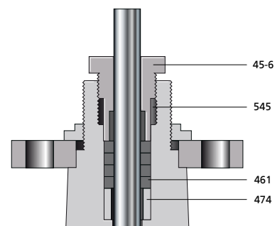
Empaquetadura del prensaestopas de grafito
