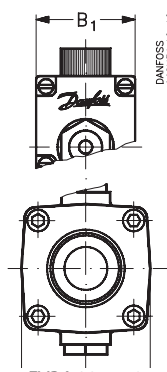
EVRA 32 et 40 Bobina con caja terminal
