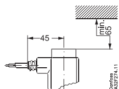
EVRA 25, 32 et 40 Bobona con cable
